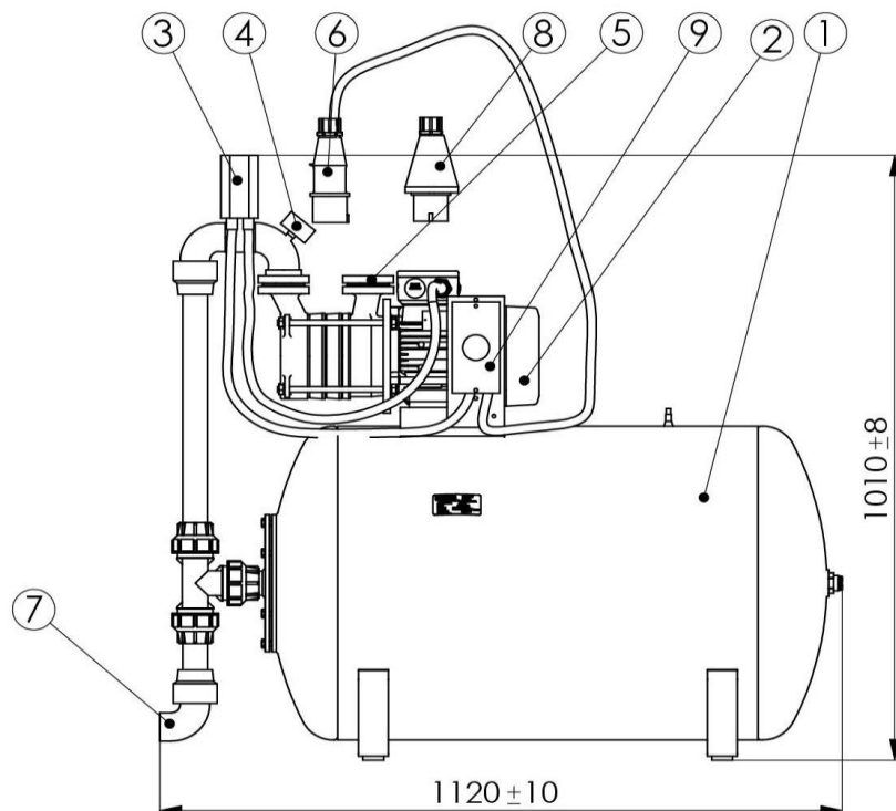
Rys. 3 Automat hydroforowy ASG.5 z pompą SM.4.02 1,5 kW/400V_Z ( Z – zabezpieczenie zwarcowe i przeciążeniowe )
