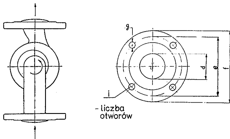
Rys. 2. Rysunek wymiarowy wraz z przekrojem
